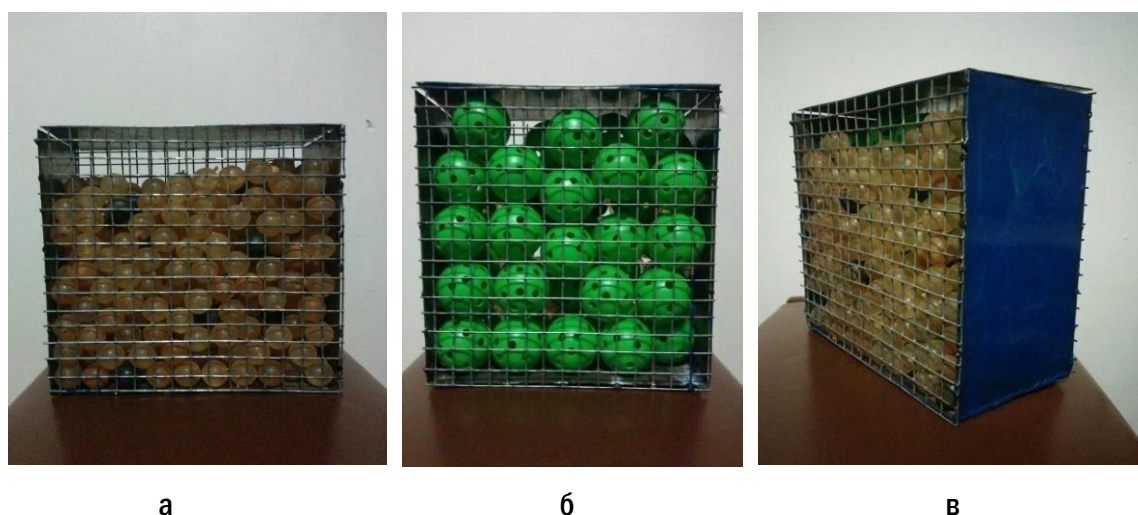
Рисунок 3. Варианты рыбозащитных кассет
