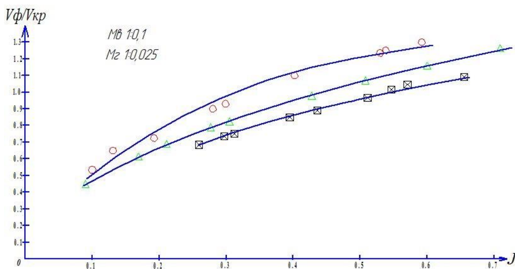
Рисунок 6. Графики зависимостей скоростей фильтрации от градиента пьезометрического напора.
