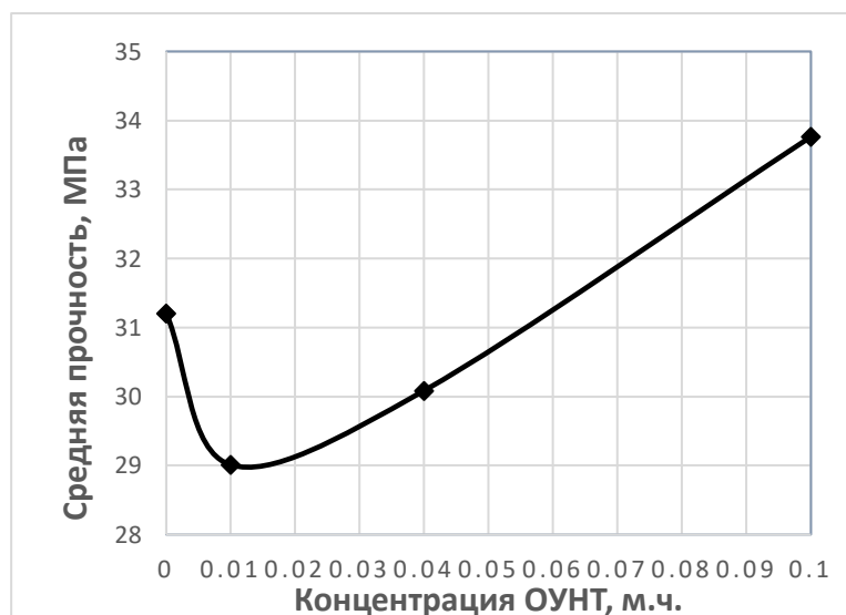
Рисунок 3. Зависимость прочности на растяжение( \sigma_p ) от содержания ОУНТ в ПВХ-композиции
