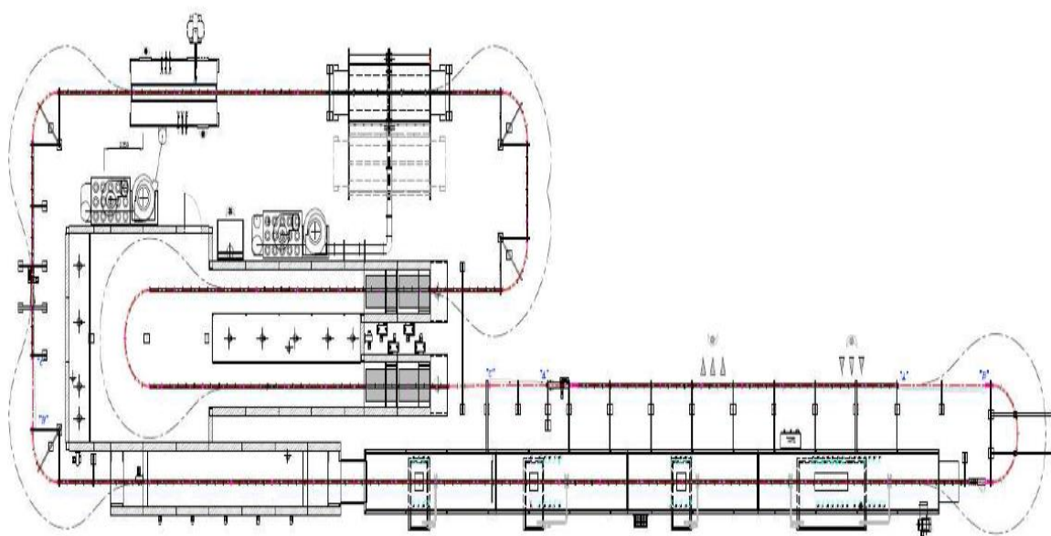
Рисунок 1. Схема размещения линии
