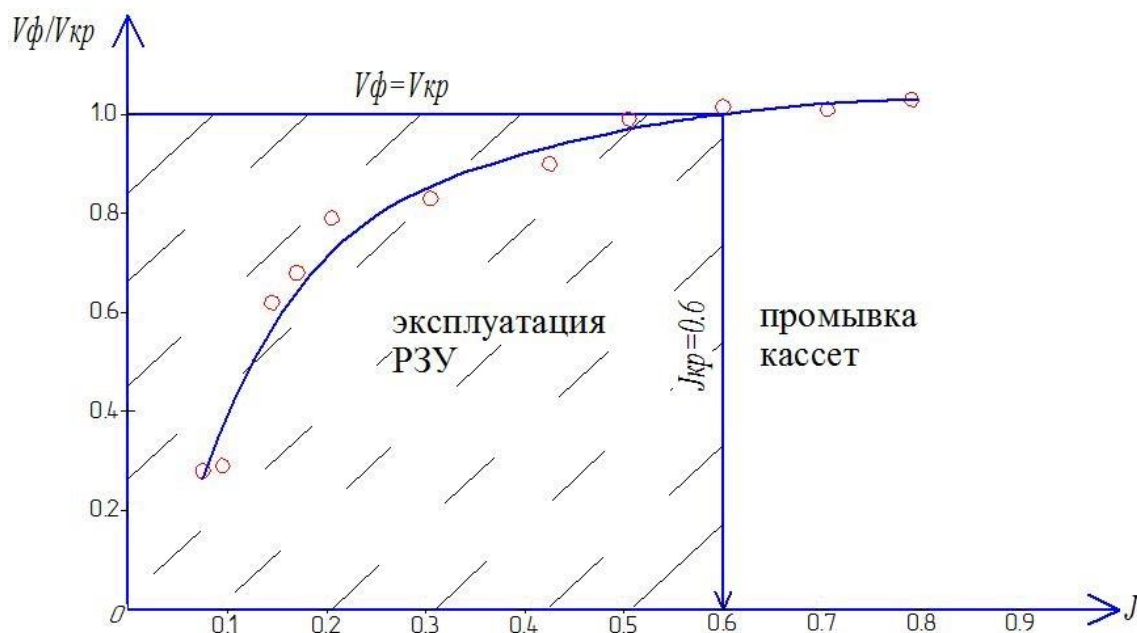
Рисунок 7. Динамика кольтации и регенерации кассеты РЗУ
