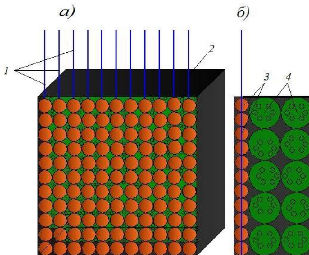
Рисунок 4. Рыбозащитная кассета со смешанным типом заполнителя:
