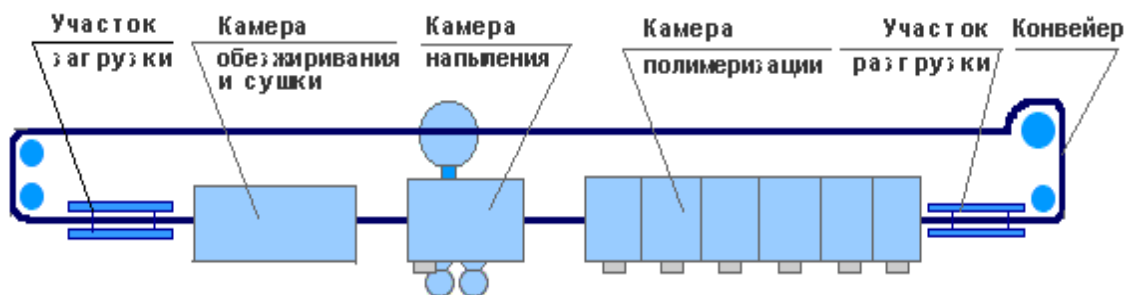
Рисунок 2. Схема конвейерной линии порошковой окраски
