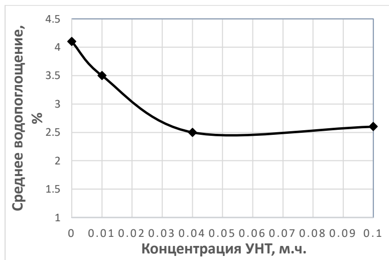
Рисунок 4. Зависимость водопоглощения (W) от содержания ОУНТ в ПВХ-композиции
