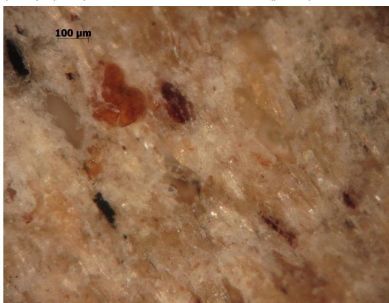
Рисунок 5. Микрофотография среза композита с 0,1% ОУНТ
