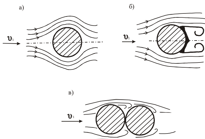
а) вязкое течение (без отрыва от струи); б) обтекание сопровождающееся отрывом потока; в) обтекание шаров, установленных вплотную друг к другу
