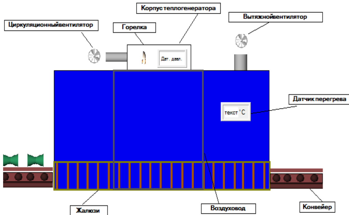
Рисунок 3. Статическая часть экрана оператора
