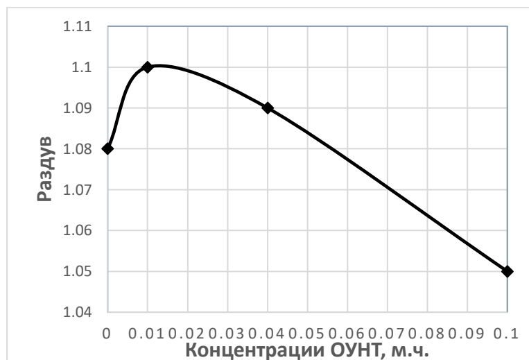
Рисунок 2. Зависимость «разбухания» экструдатов от содержания ОУНТ в ПВХ-композиции
