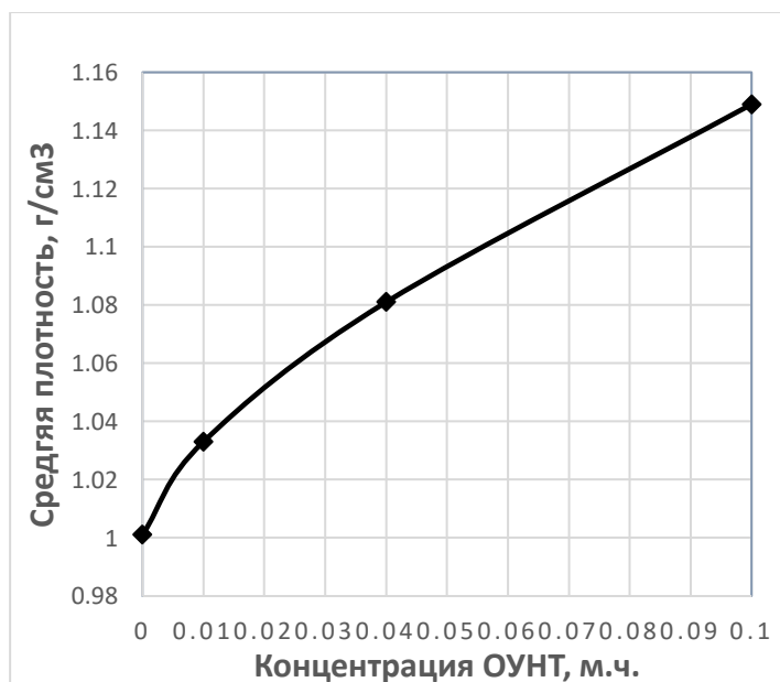
Рисунок 1. Зависимость средней плотности экструдов от содержания ОУНТ в композиции
