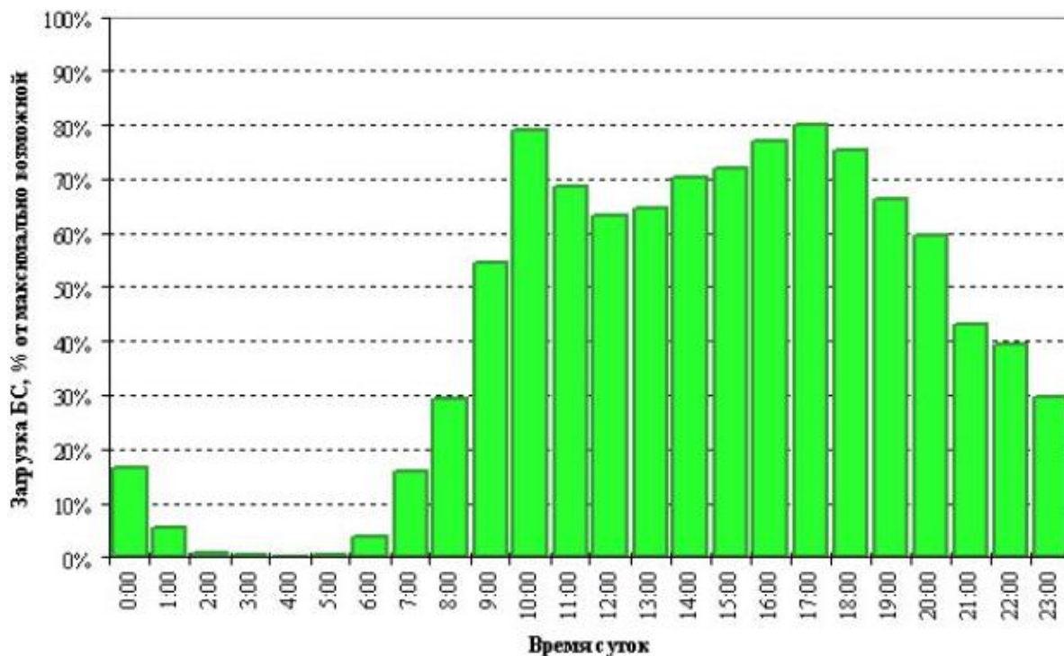
Рисунок 3. Типичный график суточной нагрузки базовой станции из [21]
