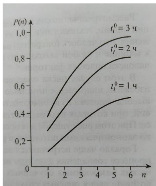
Рис. 1. Зависимость вероятностей воздействия n опасных факторов на работников на основе соотношения (2.4).
