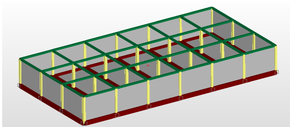
Рис. 2. Вид модель конструкции без крыши
