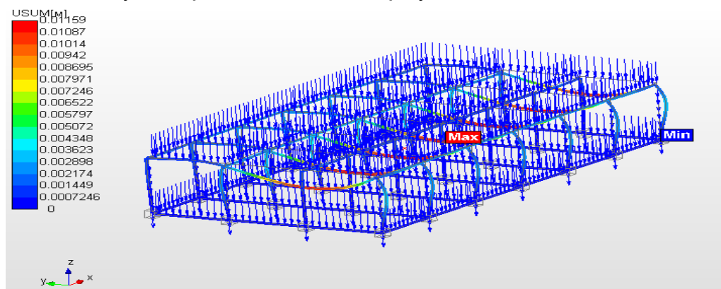
Рис. 4. Максимальное и минимальное перемещение в конструкции
