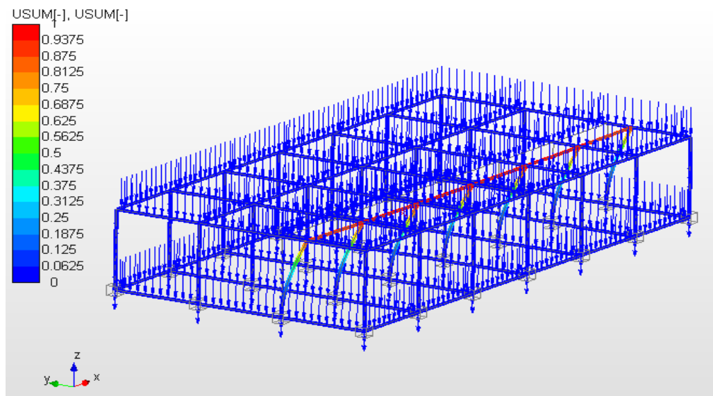
Рис. 5. Максимальный и минимальный коэффициент устойчивости конструкции
