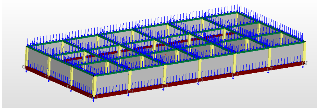
Рис. 3. Вид модели с приложенными к ней нагрузками
