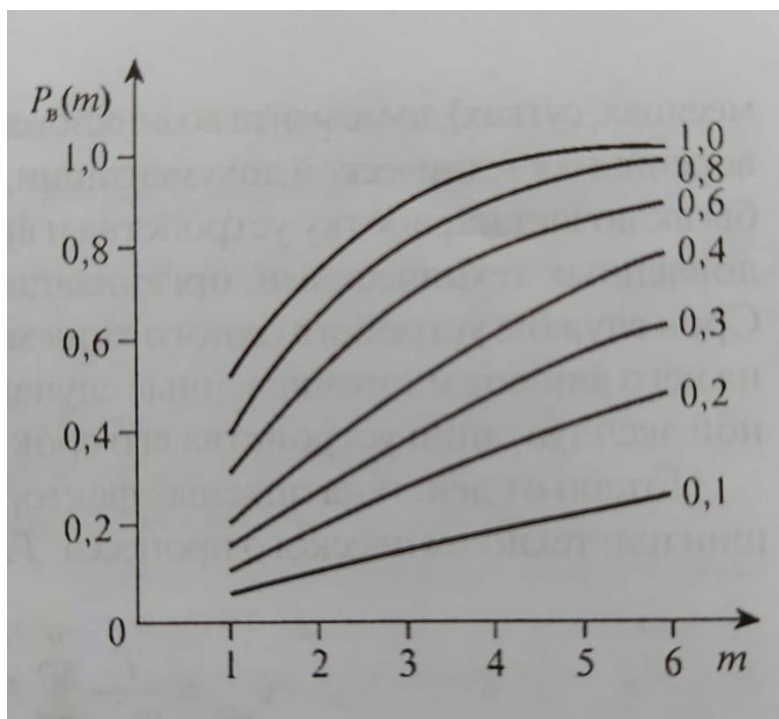
Рис. 2. Зависимость P_v(m) от m -го числа вредных факторов и d_j/D_j ( t_j^v и t_j^p – const).
