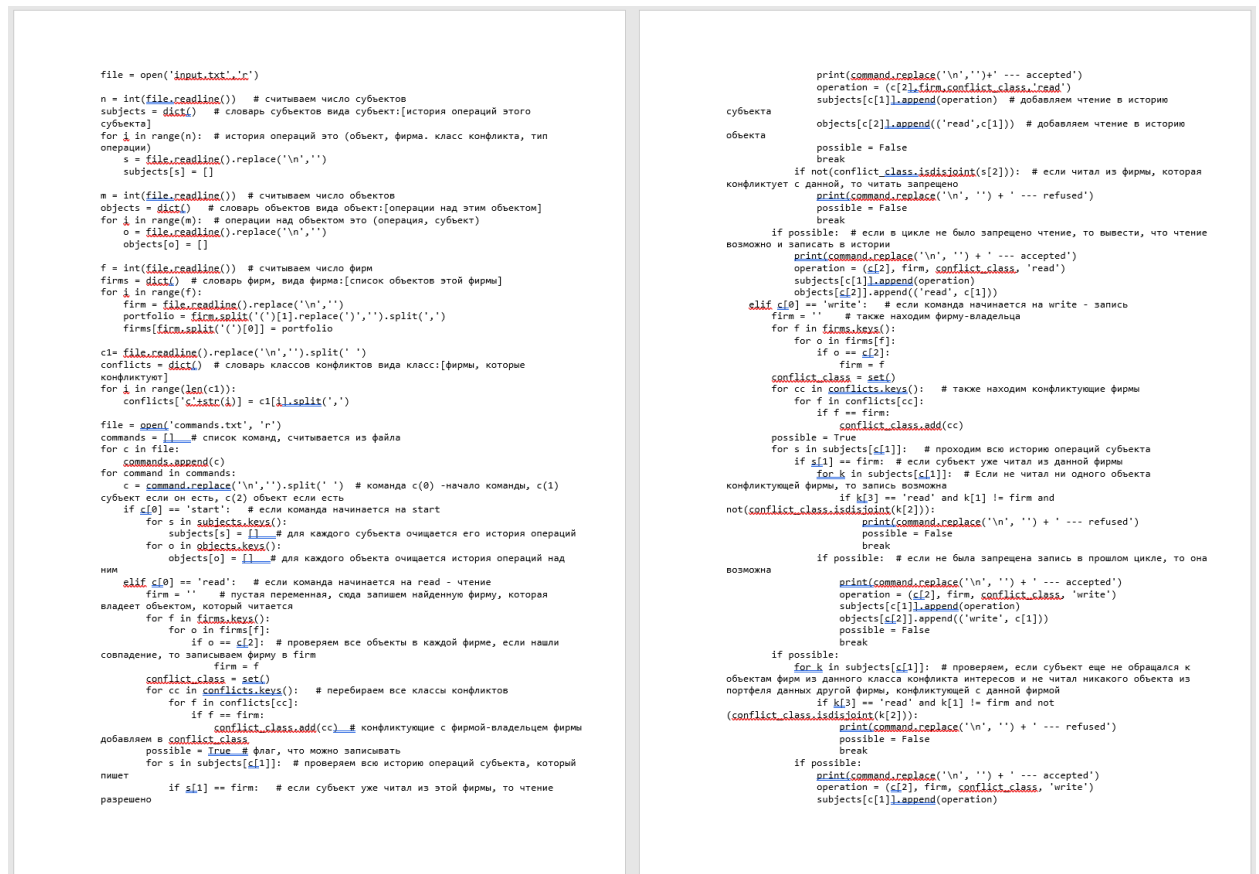
Рисунок 1. Первая и вторая часть кода разработанной решеточной модели «Китайской стены».
