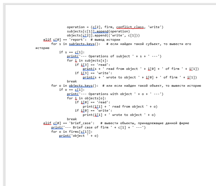
Рисунок 2. Третья часть кода разработанной решеточной модели «Китайской стены».
