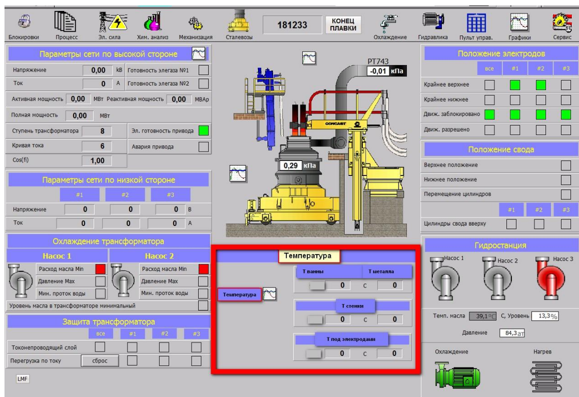
Рисунок 2. Проект внедрения дополнительных параметров в действующую SCADA-систему
