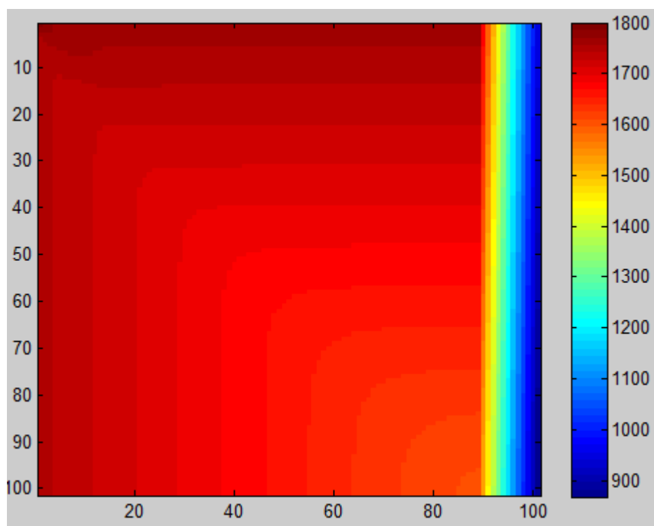
Рисунок 1. Температурное поле дуговой сталеплавильной печи
