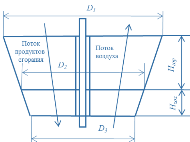
Рисунок 1. Схема вращающегося РВП с набивкой в форме усеченного конуса
