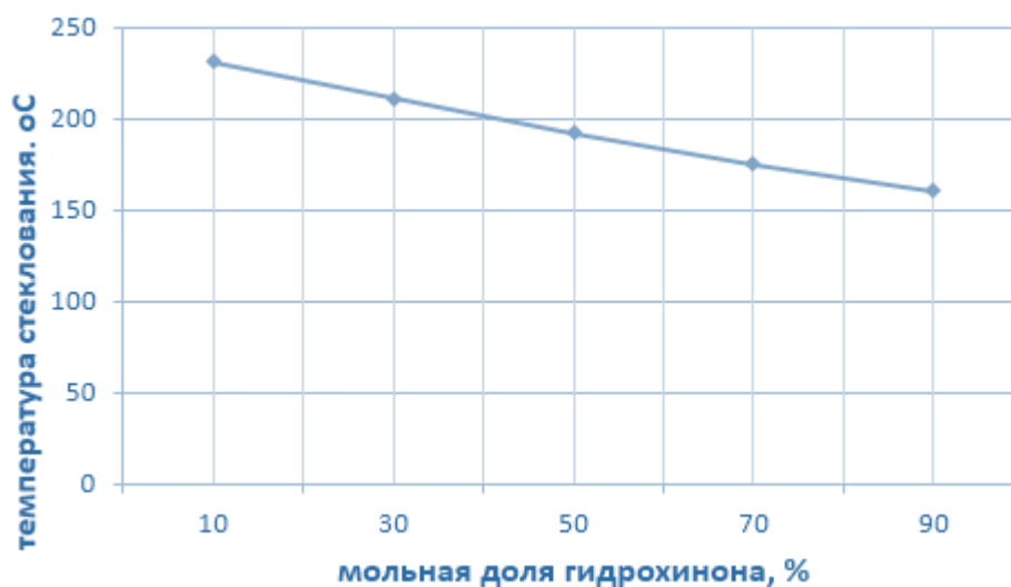
Рисунок 3. Зависимость температур стеклования сополиэфирэфиркетонов от мольной доли гидрохинона.
