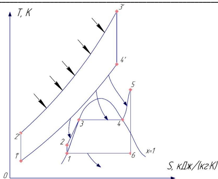
Рисунок 2. Цикл Брайтона–Ренкина ПГУ: 1'–2' – сжатие воздуха в турбокомпрессоре; 2'– 3' – подвод теплоты в камеру сгорания ГТУ; 3'– 4' – расширение продуктов сгорания в газовой турбине; 4'–1' – отвод уходящих газов; 1–2 – повышение давления питательной воды; 2–3 – нагрев питательной воды; 3–4 – процесс парообразования; 4– 5 – перегрев пара; 5–6 – процесс расширения пара; 6–1 – конденсация пара в конденсаторе
