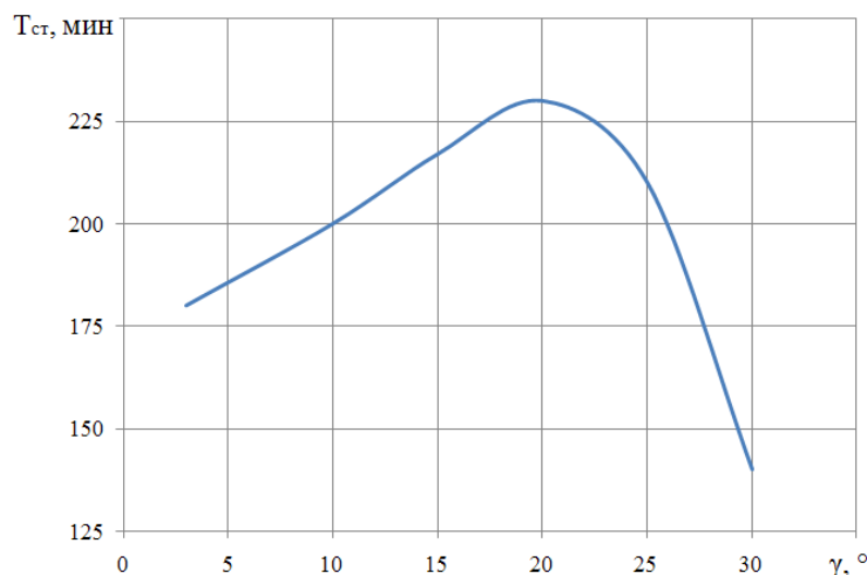
Рисунок 5. Зависимость стойкости фрезы от переднего угла
