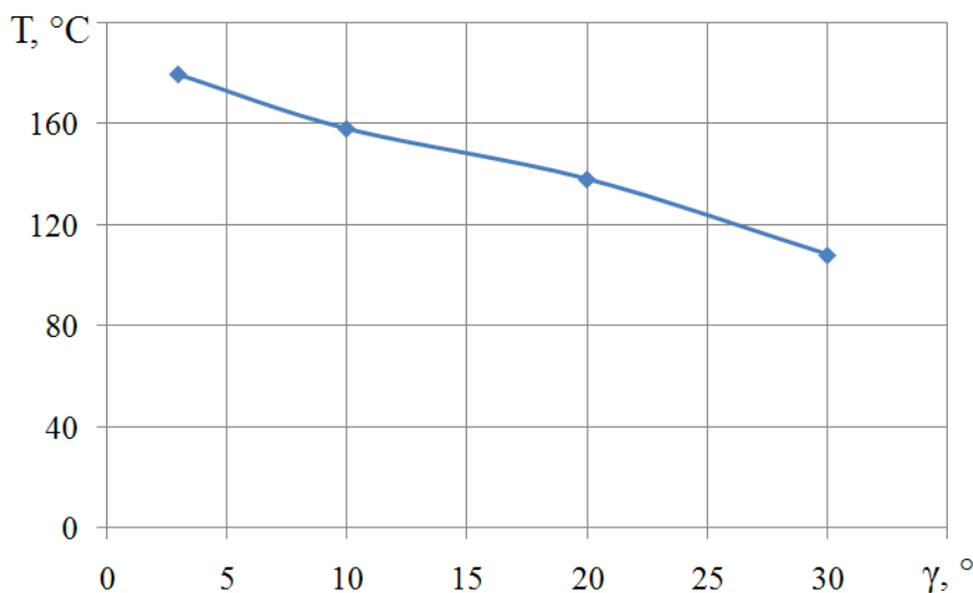
Рисунок 4. Зависимость температуры резания от переднего угла инструмента
