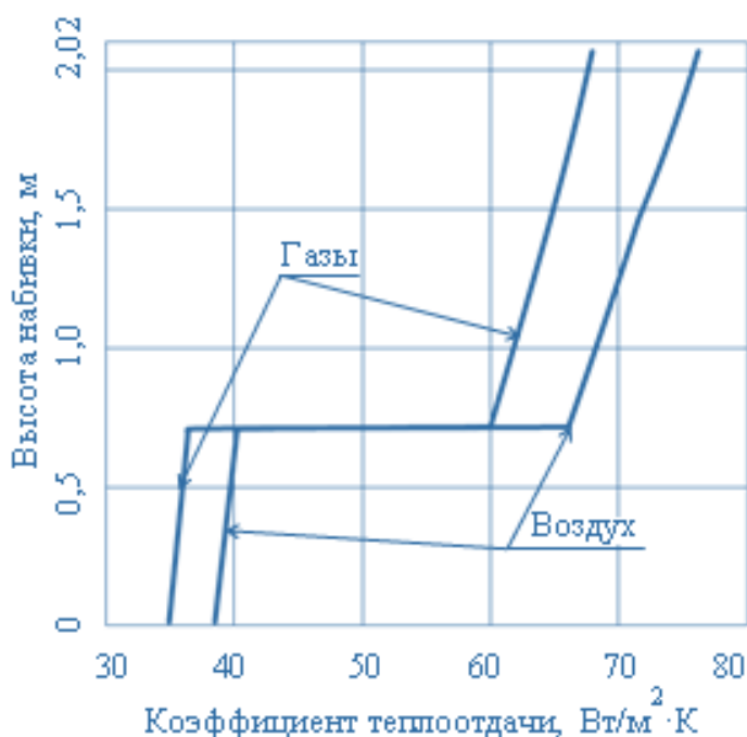
Рисунок 2. Распределение коэффициентов теплоотдачи по высоте набивки РВП-54 цилиндрической формы
