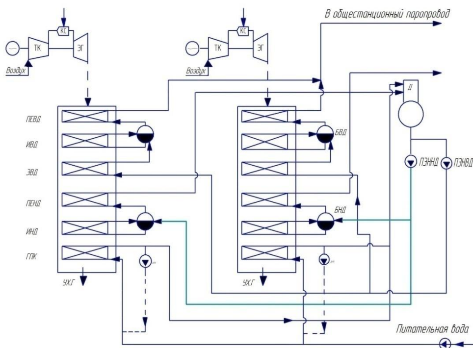
Рисунок 1. Расчетная тепловая схема ПГУ с двухконтурным котлом–утилизатором
