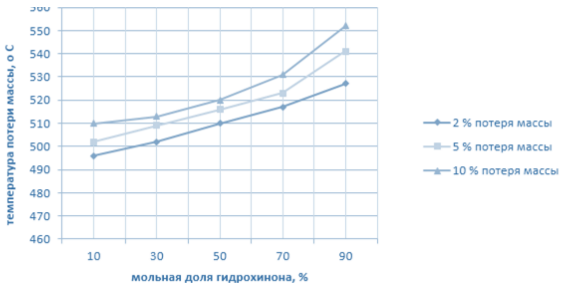
Рисунок 4. Зависимость температуры потери массы (ТГА) сополиэфирэфиркетониров от содержания гидрохинона.
