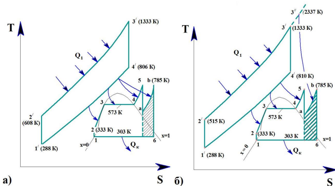
Рисунок 2. Комбинированный цикл Брайтона-Ренкина при промежуточном перегреве водяного пара в котле-утилизаторе (а) и в камере сгорания (б) ГТУ
