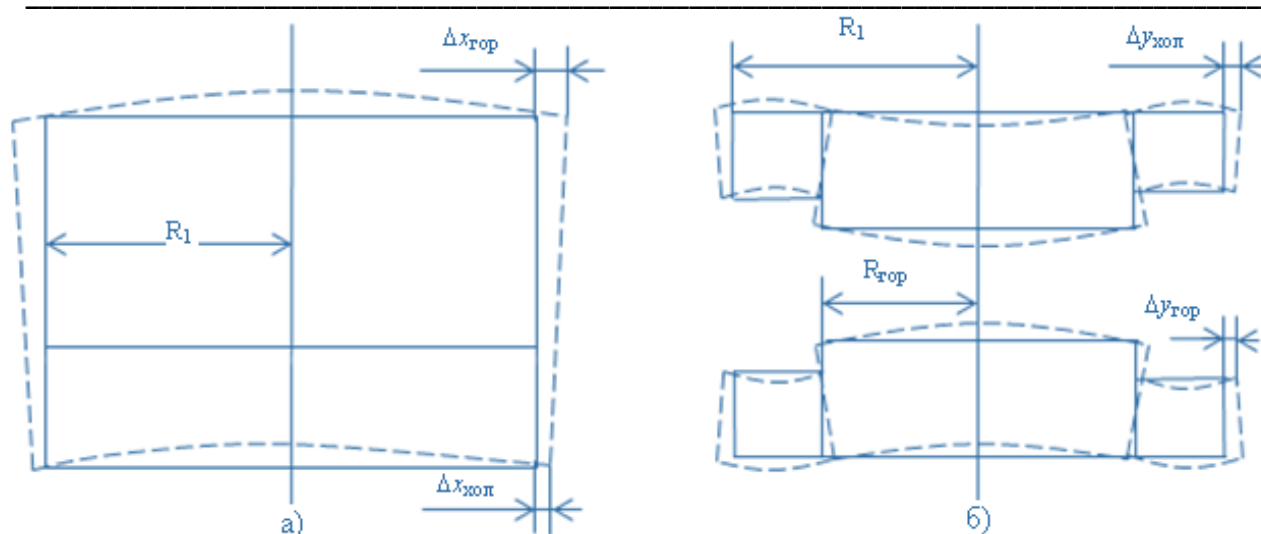
Рисунок 6. Схема температурных деформаций роторов РВП-54 цилиндрической формы (а) и двухпоточного двухходового РВП (б)
