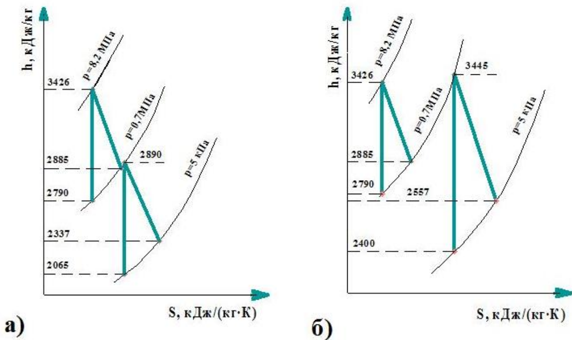
Рисунок 3. Процессы расширения водяного пара в паровой турбине К-150-8 при отсутствии (а) и с учетом вторичного перегрева (б) водяного пара в камере сгорания ГТУ
