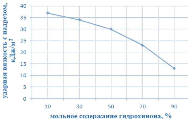
Рисунок 5. Зависимость удельной ударной вязкости сополиэфиркетониров от мольной доли гидрохинона.
