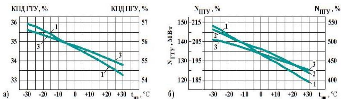
Рисунок 4. Зависимость КПД (а) и мощности (б) установок при промежуточном перегреве водяного пара в камере сгорания ГТУ от температуры наружного воздуха t_{\text{нв}} : 1 – для ГТУ, 2 – для паровой турбины, 3 – для ПГУ-450
