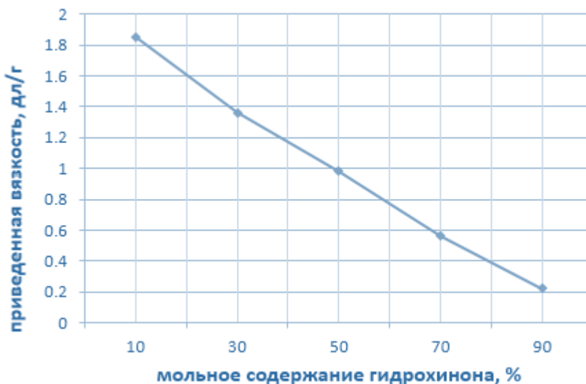
Рисунок 2. Зависимость приведенной вязкости сополиэфиркетонов от содержания гидрохинона.
