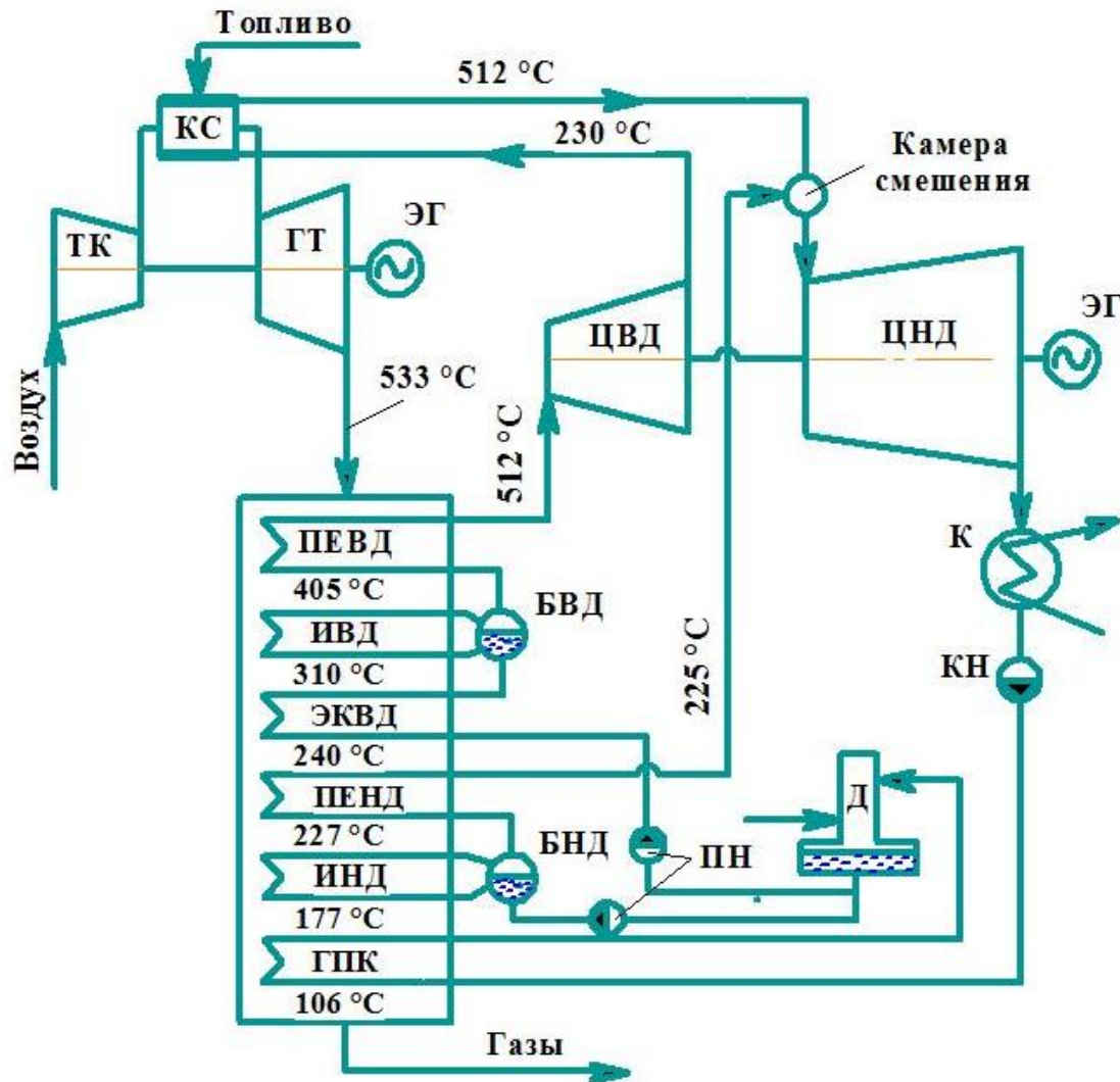
Рисунок 1. Тепловая схема ПГУ-450 с промежуточным перегревом водяного пара в камере сгорания ГТУ
