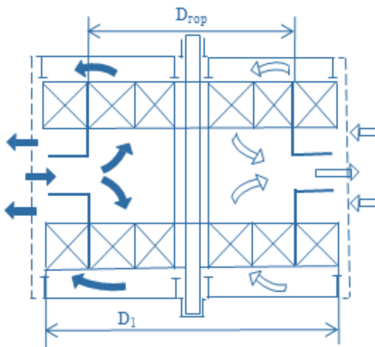
Рисунок 5. Схема двухпоточного двухходового вращающегося РВП
