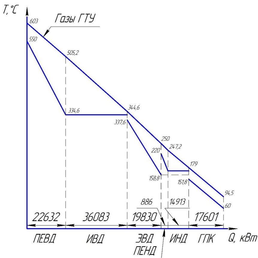
Рисунок 3. Тепловая диаграмма t=f(Q) котла-утилизатора
