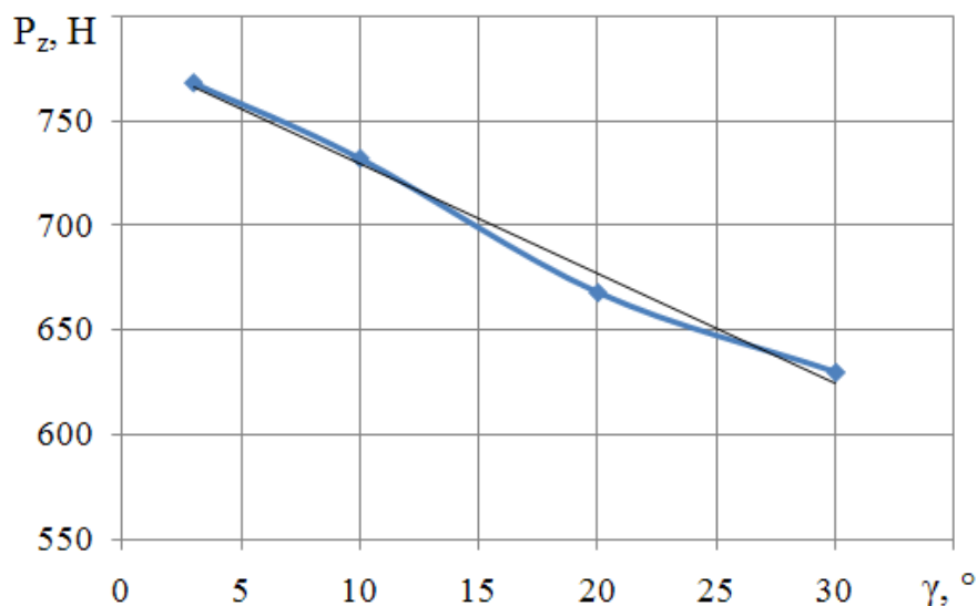
Рисунок 3. Зависимость силы резания от переднего угла инструмента
