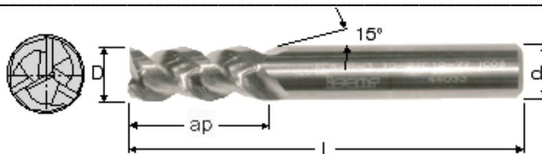
Рисунок 2. Концевая фреза Iscar Ø16 мм
