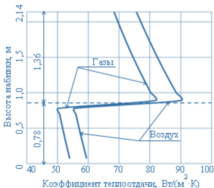
Рисунок 3. Распределение коэффициентов теплоотдачи по высоте набивки РВП-54 в форме усеченного конуса
