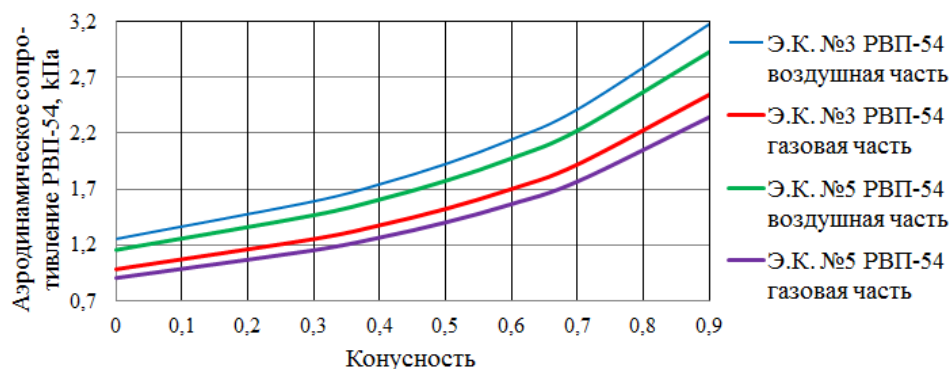
Рисунок 4. Зависимость аэродинамического сопротивления от величины конусности набивки вращающегося РВП в форме усеченного конуса
